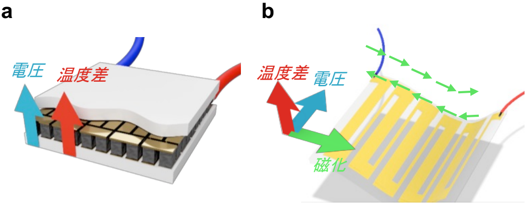
図 3 (a)従来技術（ゼーベック効果）を用いた熱電変換モジュール、(b)新技術（磁気熱電効果）を用いた無接合フレキシブル熱電変換モジュール
